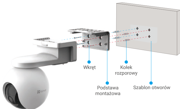
Rys. 2 Montaż ścienny
